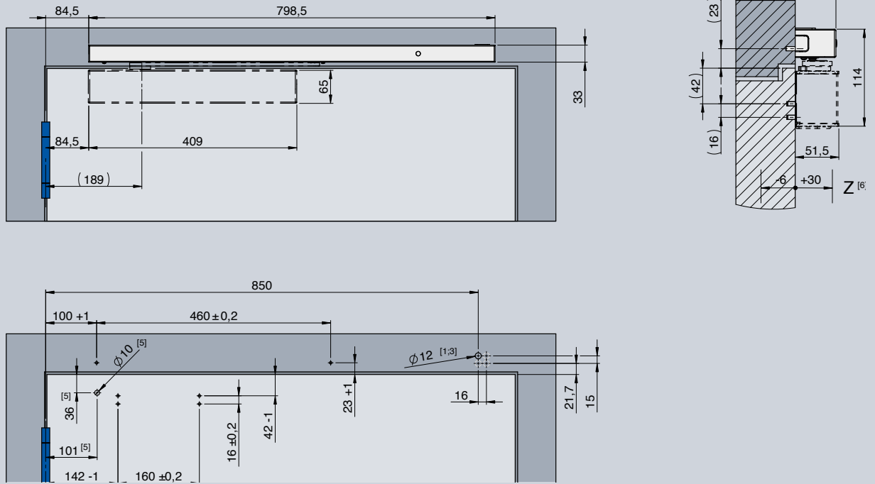
Direktmontage Gleitschiene ECO EFR III DIN-L
