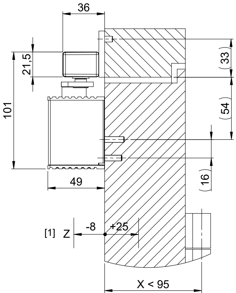
[1] Maximaler Überstand für Dickfalztüren (Z = positiv) und überstehende Zargen (Z = negativ)
